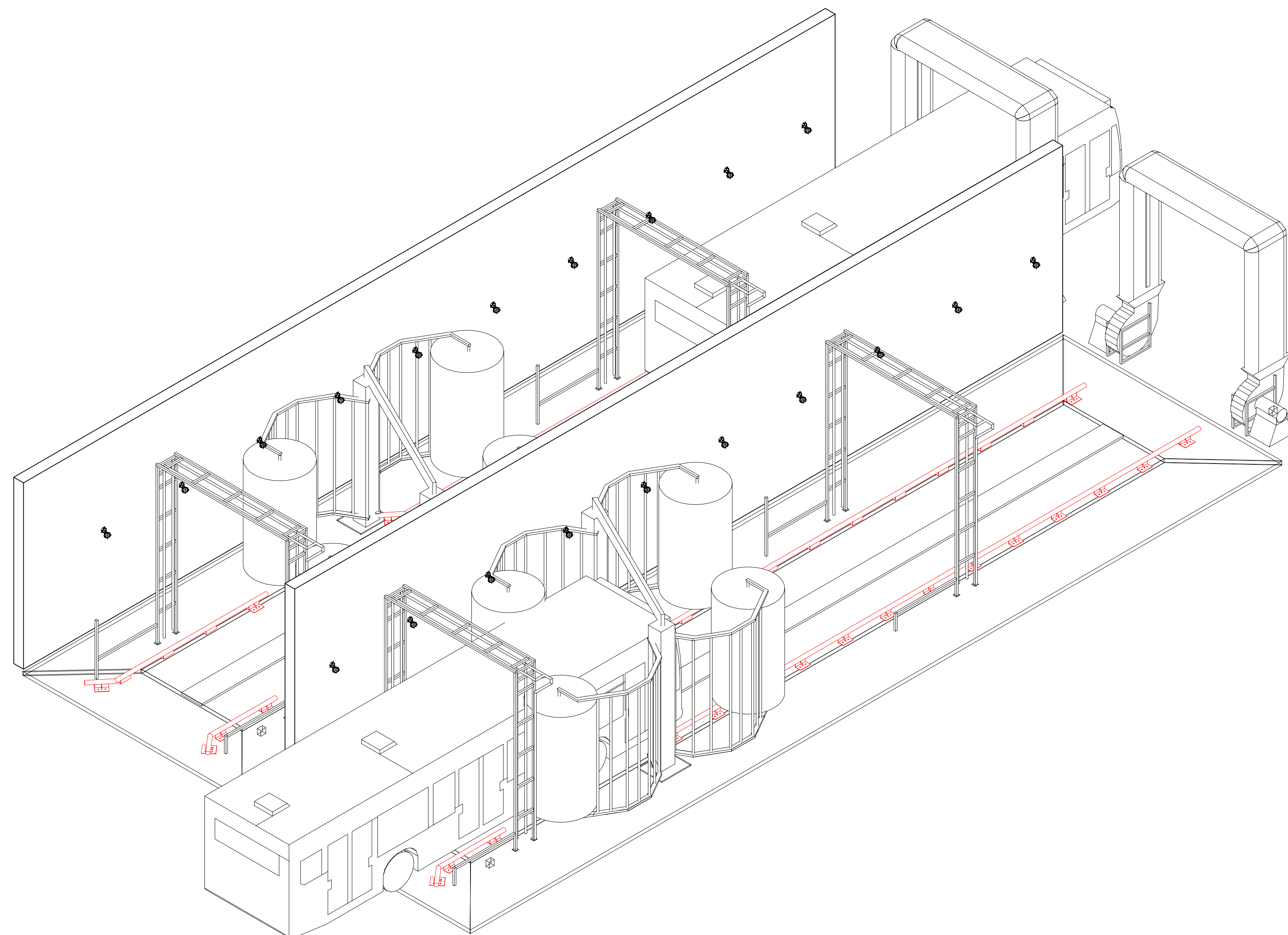
1 RIGHT SIDE ISO Scale: 3/16" = 1'-0"
